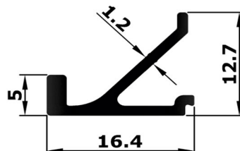
ZALI CLIP
