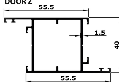
DOOR Z
