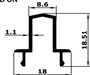
ADD ON
