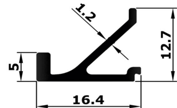
ZALI CLIP
