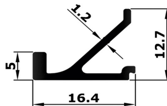
ZALI CLIP
