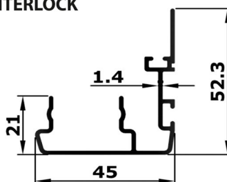
INTERLOCK
